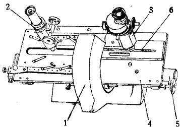
线纹比较仪外形图
